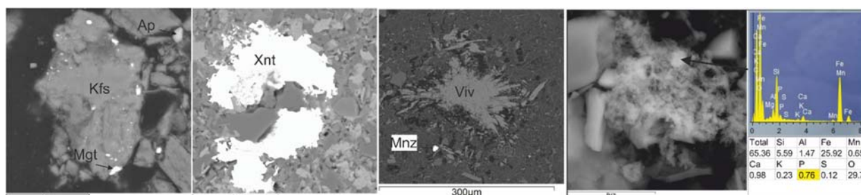
Рис. Минералы фосфора в донных отложениях Онежского озера. Символьные обозначение минералов: Xtm – ксенотим; Mnz– монацит; Mgt –магнетит; Kfs– К-полевоы шпат; Ap –апатит; Viv– вивианит
