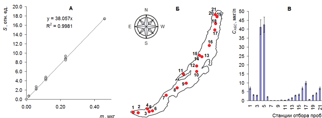
Рис. A – калибровочная зависимость площади пиков S от суммарного содержания метиловых эфиров алкилбензолсульфокислот в калибровочных растворах; B – схема станций отбора проб снега со льда оз. Байкал в марте 2022 г.; В – концентрации линейных алкилбензолсульфонатов натрия ( C_{\text{АБС}} , мкг/л) в снеговой воде
