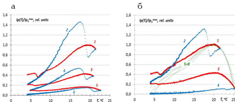
Рис. Зависимость интенсивности свечения воды р. Ангары от температуры.
